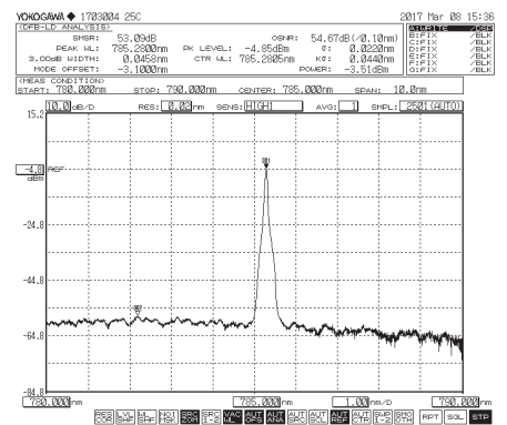
785nm
